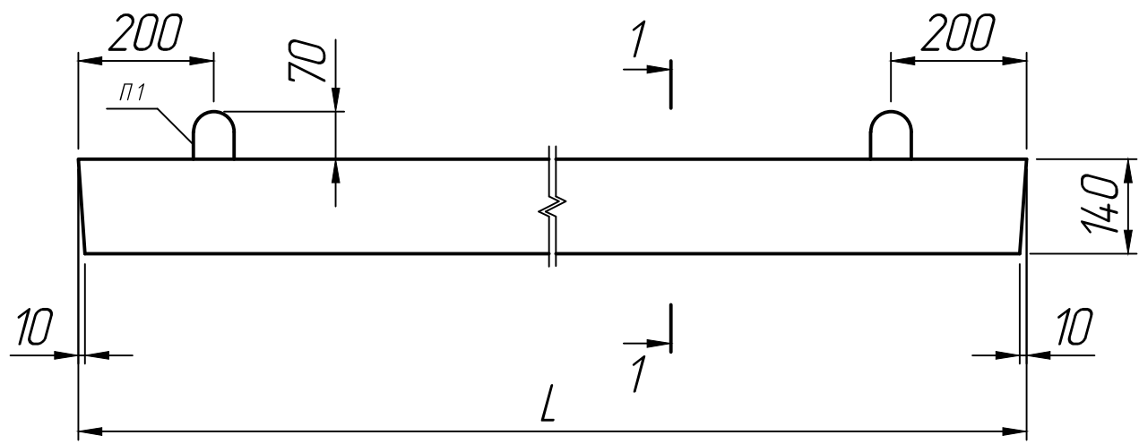
Размеры, мм
