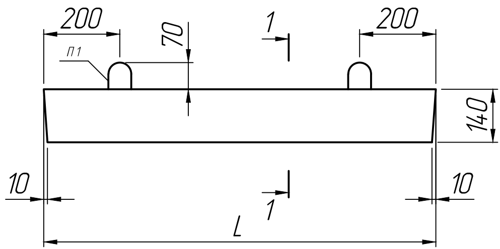
Размеры, мм
