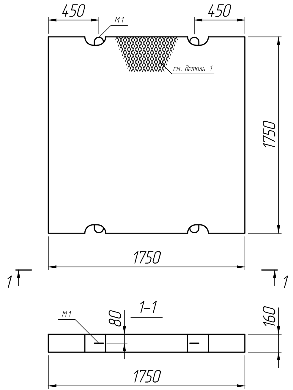
1 - деталь рифления на рабочей поверхности плиты
