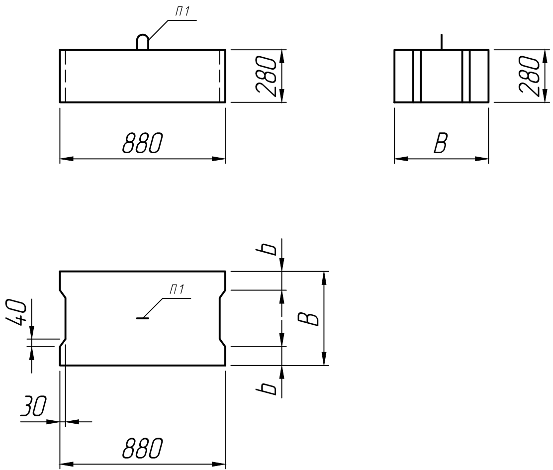
Размеры, мм
