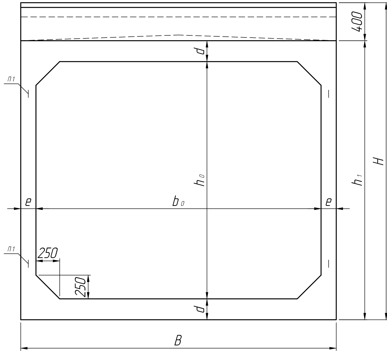
Размеры, мм
