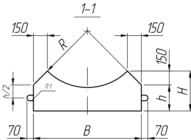
Размеры, мм
